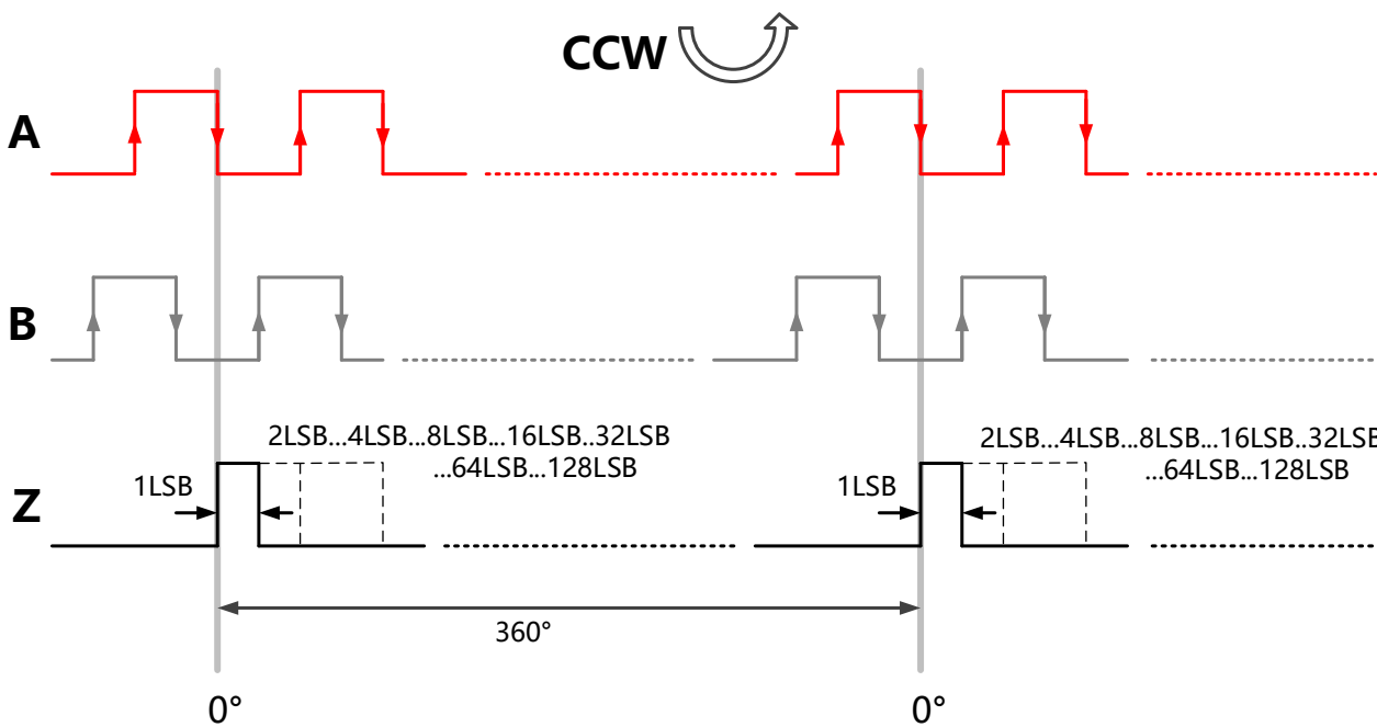
图-10: Z信号宽度=1、2、4、8、16、32、64、128LSBs示意图
