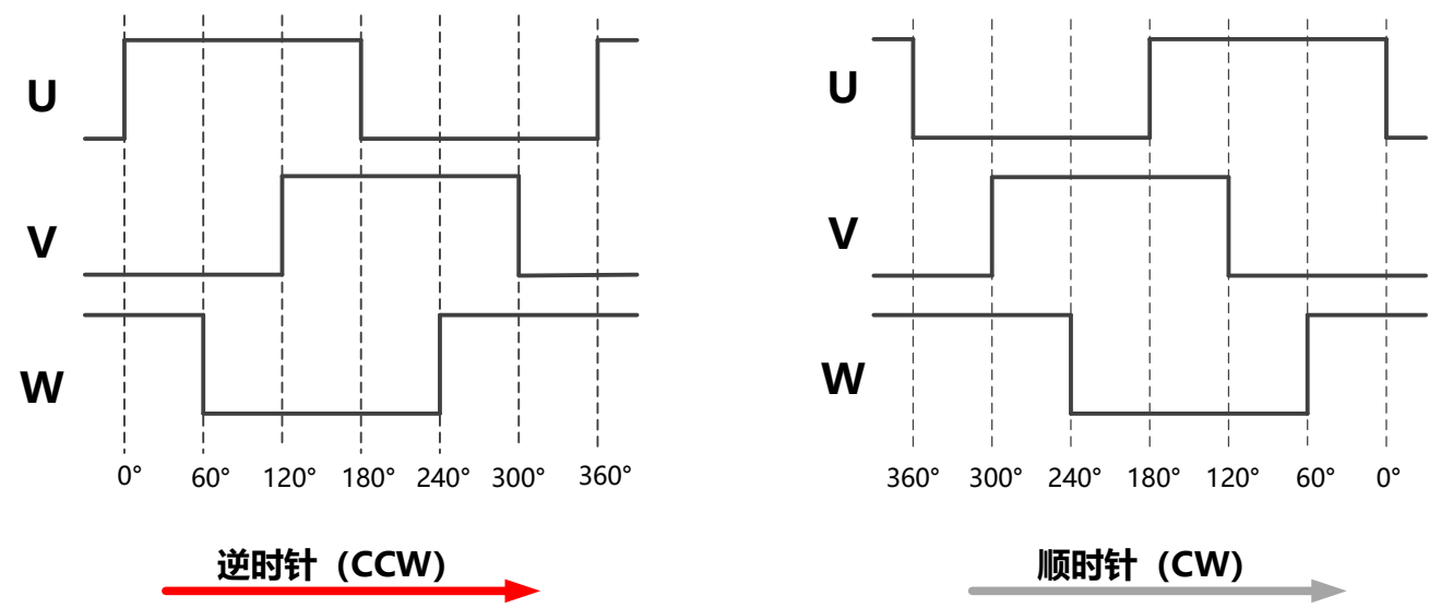
图-14: UVW输出波形
