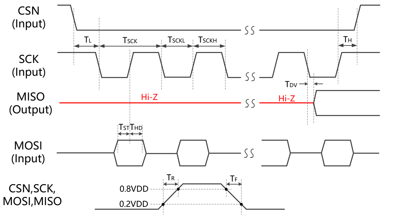
图-17: SPI时序图
