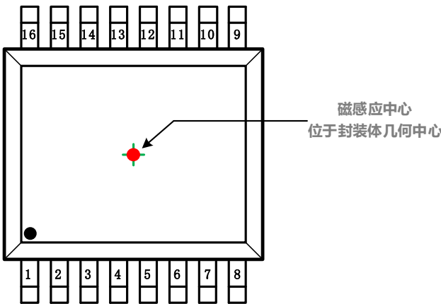
图-1: MT6826S TSSOP-16封装外观图
