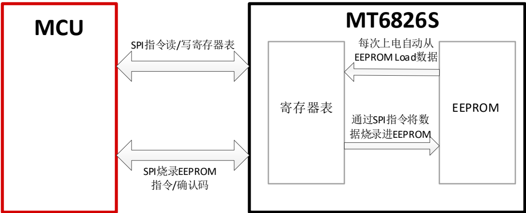
图-22: 寄存器表和EEPROM关系
