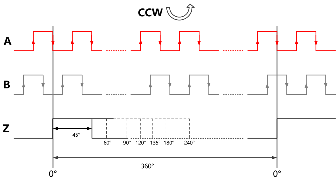
图-11: Z信号宽度=45°、60°、90°、120°、135°、180°、240°示意图
